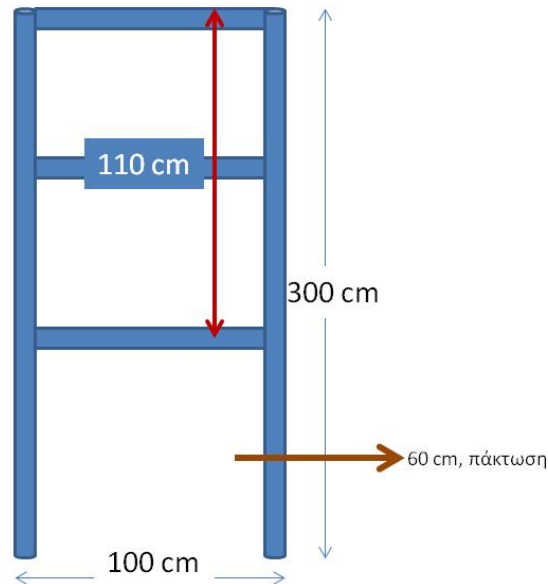
Σκελετός τύπου 2
