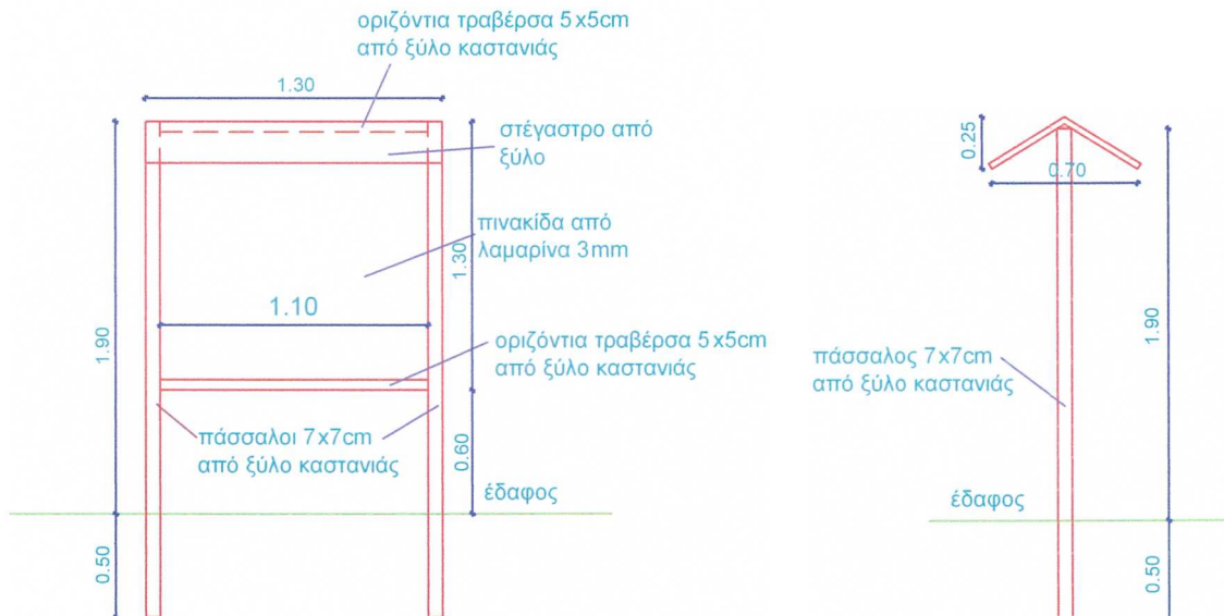
ΕΙΚΟΝΑ 1. ΟΨΗ-ΤΟΜΗ ΠΙΝΑΚΙΔΑΣ
